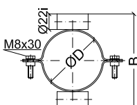
Статическое распорное кольцо для регулируемого отвода 19
